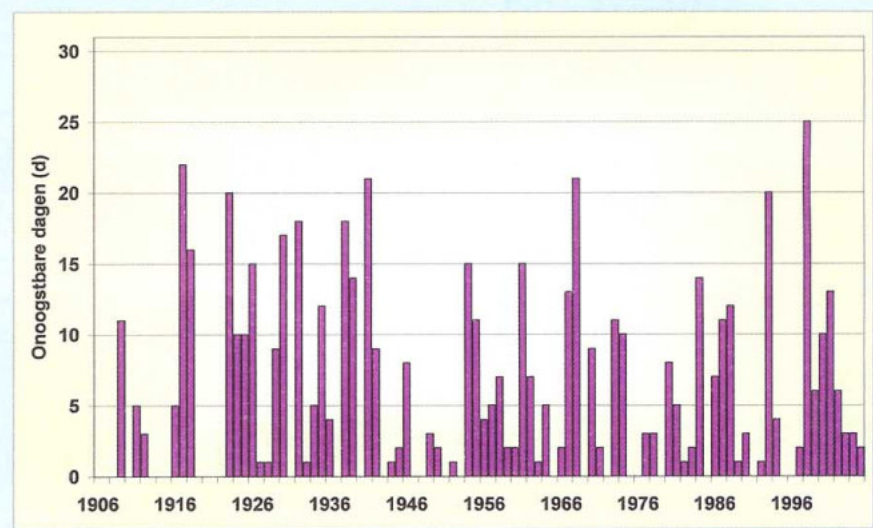
Afb. 4: Onoogstbare dagen voor de overgedimensioneerde afwatering, uitgedrukt als dagen in oktober met een drukhoogte in de bovengrond groter dan -50 cm.
