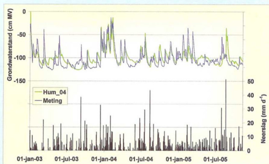
Afb. 1: Gemeten en gesimuleerde grondwaterstanden.
