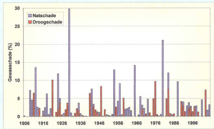
Afb. 3: Droogte- en natschade door verminderde gewasgroei voor de NBW-norm.
